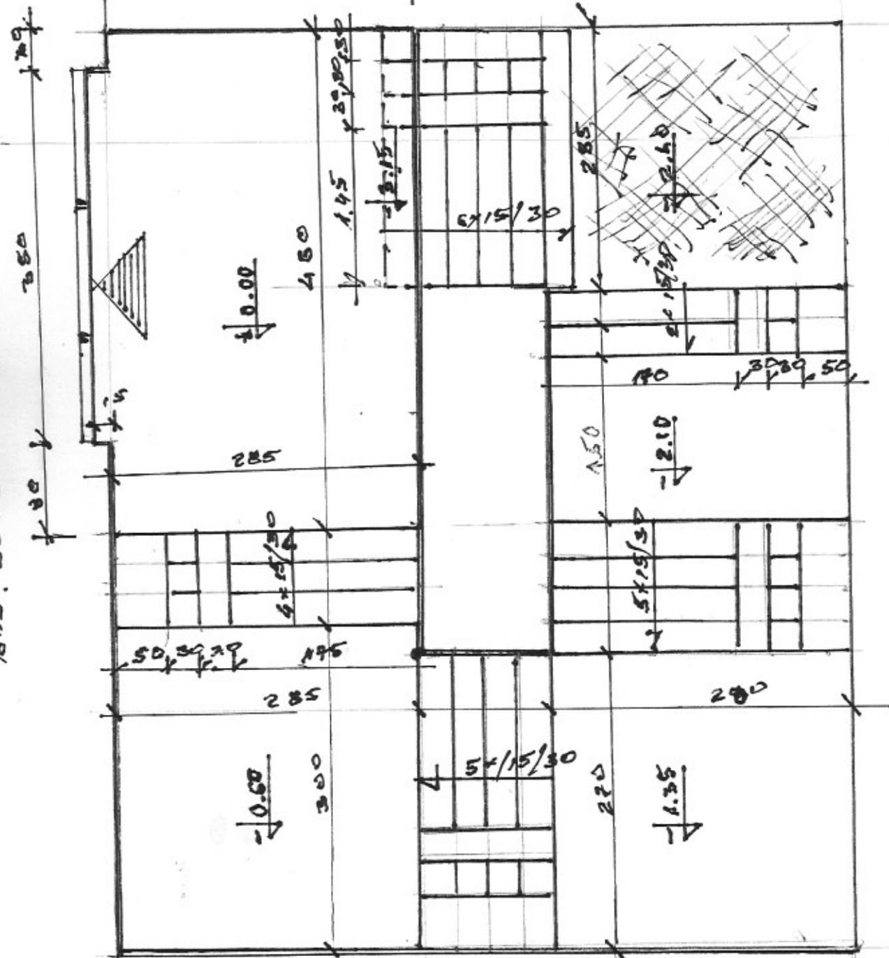
RZUT SCHODÓW
