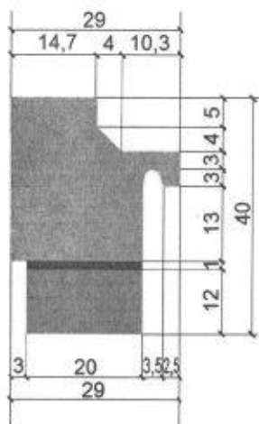
PRZEKRÓJ BORTNICY
