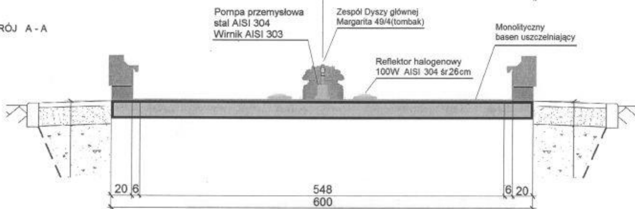
PRZEKRÓJ BORTNICY
